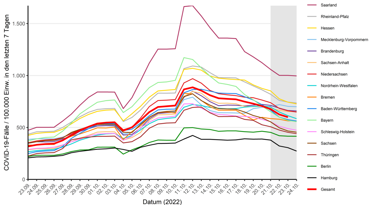
Abbildung 2: Darstellung der übermittelten COVID-19-Fälle/100.000 Einwohner über 7 Tage in Deutschland nach Bundesland und Meldedatum in den Gesundheitsämtern (24.10.2022, 0:00 Uhr). Für den grau markierten Bereich ist in den Folgetagen noch mit nachübermittelten Fällen und damit mit einer Erhöhung der Inzidenz zu rechnen.
