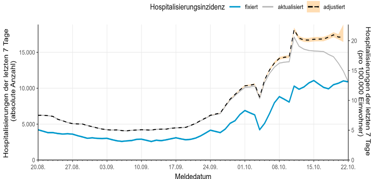
Abbildung 3: Darstellung der hospitalisierten COVID-19-Fälle/100.000 Einwohner über 7 Tage in Deutschland nach Meldedatum (24.10.2022, 0:00 Uhr). Die tagesaktuell berichtete Hospitalisierungsinzidenz (fixiert) wird in blau, mit Berücksichtigung der verzögert berichteten Hospitalisierungen (aktualisiert) in grau dargestellt. Die Schätzung der zu erwartenden Anzahl an verzögert berichteten Hospitalisierungen wird als gestrichelte Linie mit 95%-Prädiktionsintervall (in orange) gezeigt. Die Skalen geben die jeweilige absolute Anzahl (y-Achse, links) und den Anteil pro 100.000 Einw. (y-Achse, rechts) an.
