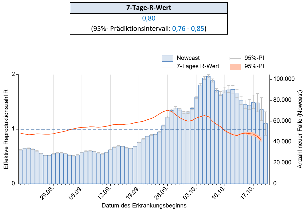
Abbildung 4: Darstellung des geschätzten R-Werts (in orange) in den letzten 60 Tagen, vor dem Hintergrund der durch das Nowcasting geschätzten Fallzahlen nach Erkrankungsbeginn (Stand 24.10.2022, 0:00 Uhr, unter Berücksichtigung der Fälle mit Erkrankungsbeginn bis 20.10.2022).
