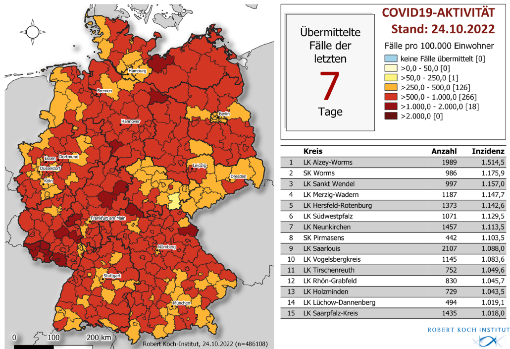
Abbildung 1: An das RKI übermittelte COVID-19-Fälle mit einem Meldedatum innerhalb der letzten 7 Tage in Deutschland nach Kreis und Bundesland (n = 486.108, 24.10.2022, 0:00 Uhr). Die Fälle werden in der Regel nach dem Kreis ausgewiesen, aus dem sie übermittelt wurden. Dies entspricht in der Regel dem Wohnort. Wohnort und wahrscheinlicher Infektionsort müssen nicht übereinstimmen.
