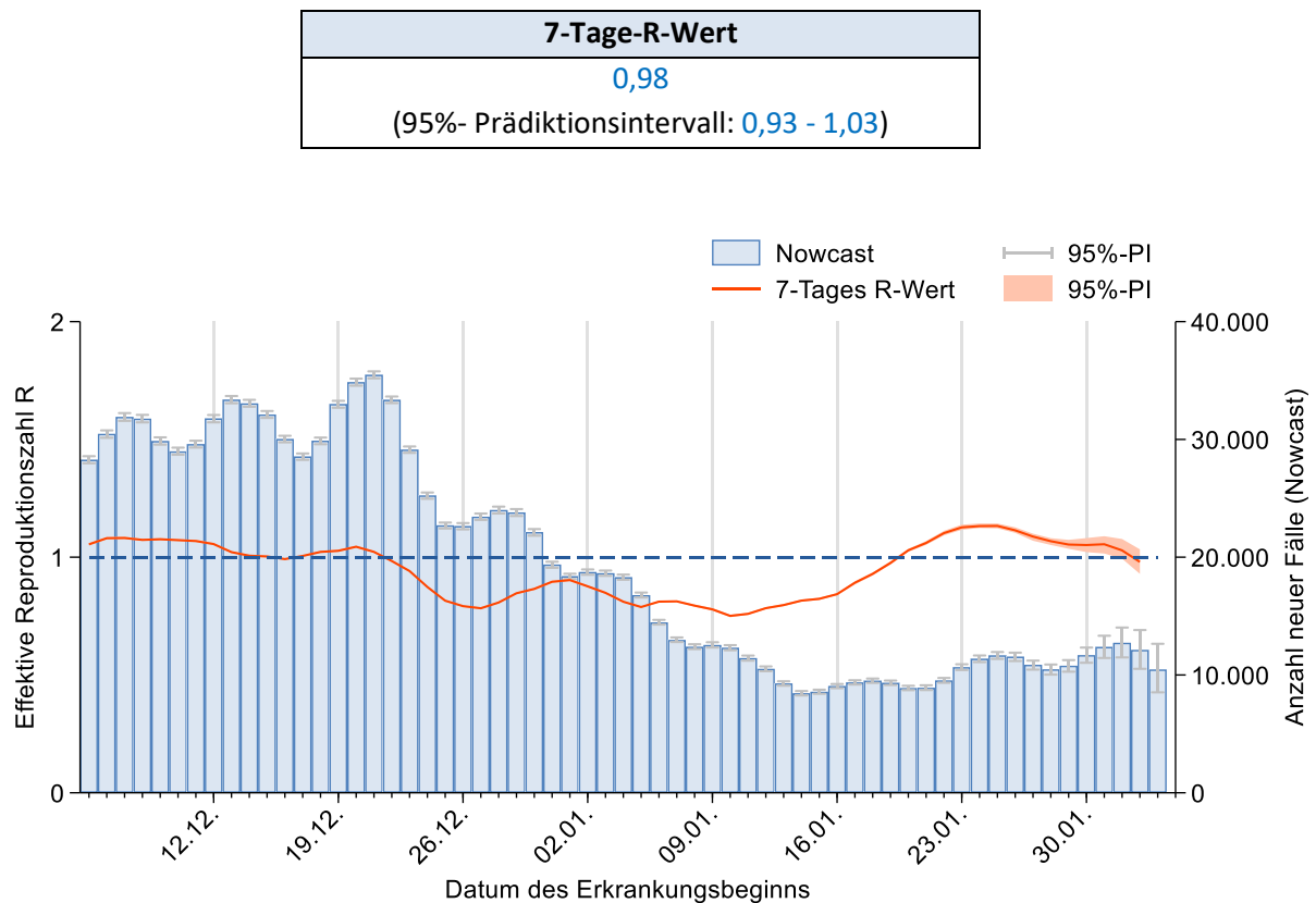
Abbildung 4: Darstellung des geschätzten R-Werts (in orange) in den letzten 60 Tagen, vor dem Hintergrund der durch das Nowcasting geschätzten Fallzahlen nach Erkrankungsbeginn (Stand 07.02.2023, 0:00 Uhr, unter Berücksichtigung der Fälle mit Erkrankungsbeginn bis 03.02.2023).
