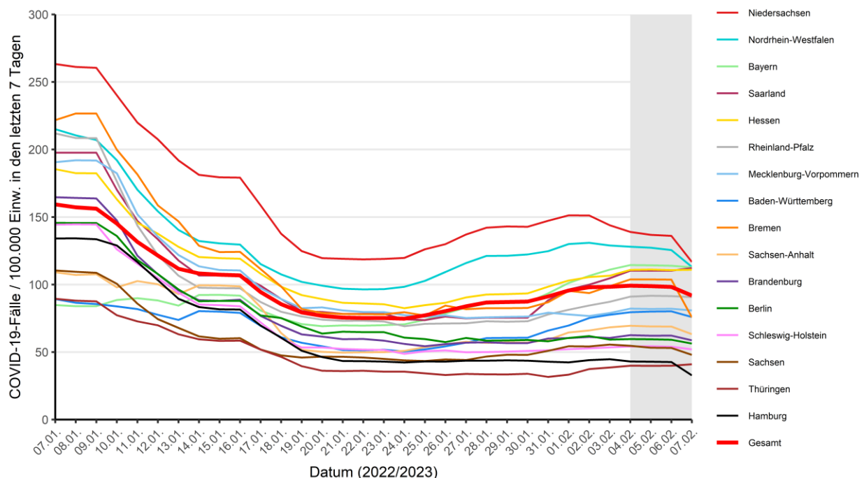
Abbildung 2: Darstellung der übermittelten COVID-19-Fälle/100.000 Einwohner über 7 Tage in Deutschland nach Bundesland und Meldedatum in den Gesundheitsämtern (07.02.2023, 0:00 Uhr). Für den grau markierten Bereich ist in den Folgetagen noch mit nachübermittelten Fällen und damit mit einer Erhöhung der Inzidenz zu rechnen.
