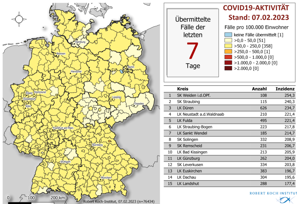
Abbildung 1: An das RKI übermittelte COVID-19-Fälle mit einem Meldedatum innerhalb der letzten 7 Tage in Deutschland nach Kreis und Bundesland (n = 76.434, 07.02.2023, 0:00 Uhr). Die Fälle werden in der Regel nach dem Kreis ausgewiesen, aus dem sie übermittelt wurden. Dies entspricht in der Regel dem Wohnort. Wohnort und wahrscheinlicher Infektionsort müssen nicht übereinstimmen.
