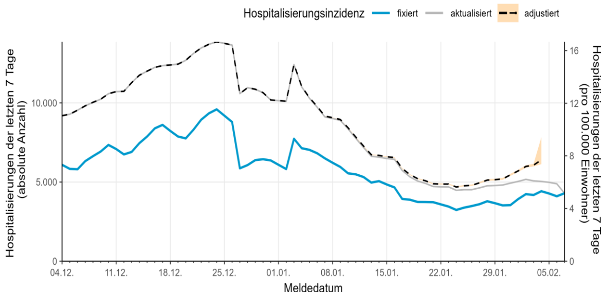
Abbildung 3: Darstellung der hospitalisierten COVID-19-Fälle/100.000 Einwohner über 7 Tage in Deutschland nach Meldedatum (07.02.2023, 0:00 Uhr). Die tagesaktuell berichtete Hospitalisierungsinzidenz (fixiert) wird in blau, mit Berücksichtigung der verzögert berichteten Hospitalisierungen (aktualisiert) in grau dargestellt. Die Schätzung der zu erwartenden Anzahl an verzögert berichteten Hospitalisierungen wird als gestrichelte Linie mit 95%-Prädiktionsintervall (in orange) gezeigt. Die Skalen geben die jeweilige absolute Anzahl (y-Achse, links) und den Anteil pro 100.000 Einw. (y-Achse, rechts) an.
