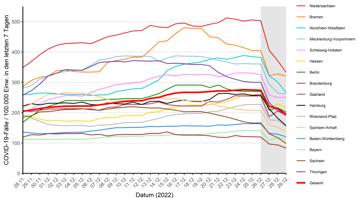
Abbildung 2: Darstellung der übermittelten COVID-19-Fälle/100.000 Einwohner über 7 Tage in Deutschland nach Bundesland und Meldedatum in den Gesundheitsämtern (29.12.2022, 0:00 Uhr). Für den grau markierten Bereich ist in den Folgetagen noch mit nachübermittelten Fällen und damit mit einer Erhöhung der Inzidenz zu rechnen.
