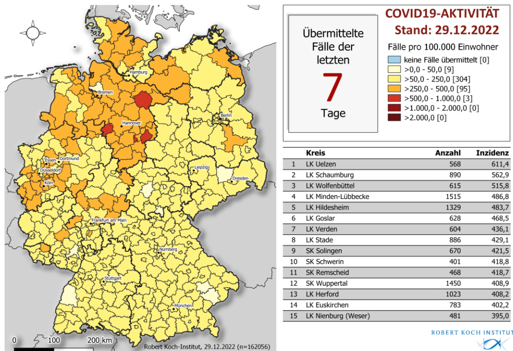
Abbildung 1: An das RKI übermittelte COVID-19-Fälle mit einem Meldedatum innerhalb der letzten 7 Tage in Deutschland nach Kreis und Bundesland (n = 162.056, 29.12.2022, 0:00 Uhr). Die Fälle werden in der Regel nach dem Kreis ausgewiesen, aus dem sie übermittelt wurden. Dies entspricht in der Regel dem Wohnort. Wohnort und wahrscheinlicher Infektionsort müssen nicht übereinstimmen.
