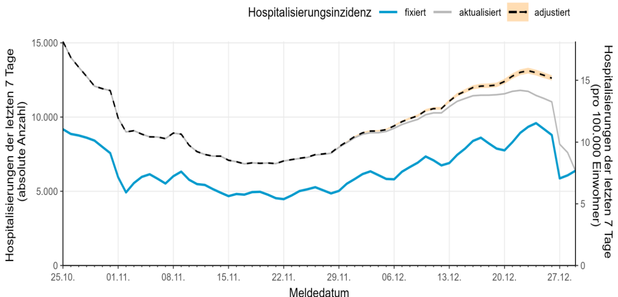
Abbildung 3: Darstellung der hospitalisierten COVID-19-Fälle/100.000 Einwohner über 7 Tage in Deutschland nach Meldedatum (29.12.2022, 0:00 Uhr). Die tagesaktuell berichtete Hospitalisierungsinzidenz (fixiert) wird in blau, mit Berücksichtigung der verzögert berichteten Hospitalisierungen (aktualisiert) in grau dargestellt. Die Schätzung der zu erwartenden Anzahl an verzögert berichteten Hospitalisierungen wird als gestrichelte Linie mit 95%-Prädiktionsintervall (in orange) gezeigt. Die Skalen geben die jeweilige absolute Anzahl (y-Achse, links) und den Anteil pro 100.000 Einw. (y-Achse, rechts) an.
