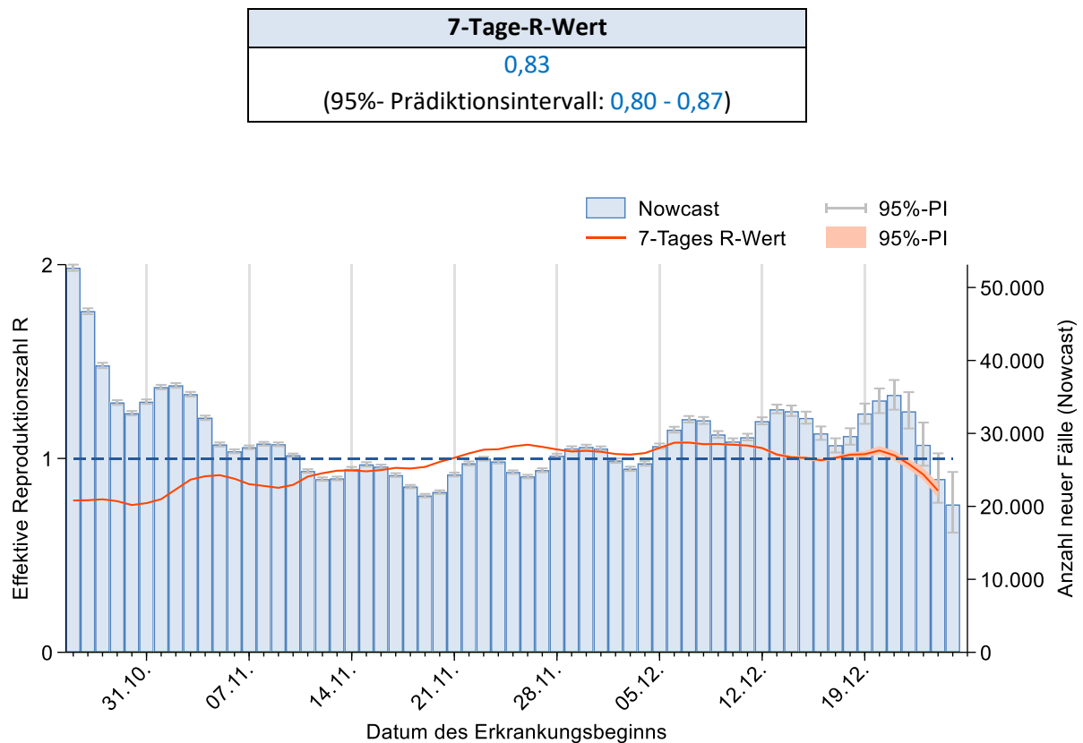
Abbildung 4: Darstellung des geschätzten R-Werts (in orange) in den letzten 60 Tagen, vor dem Hintergrund der durch das Nowcasting geschätzten Fallzahlen nach Erkrankungsbeginn (Stand 29.12.2022, 0:00 Uhr, unter Berücksichtigung der Fälle mit Erkrankungsbeginn bis 25.12.2022).
