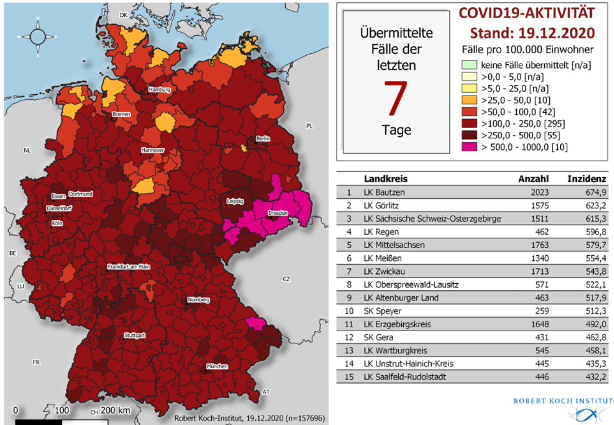
Abbildung 1: An das RKI übermittelte COVID-19-Fälle mit einem Meldedatum innerhalb der letzten 7 Tage in Deutschland nach Kreis und Bundesland (n = 157.696, 19.12.2020, 0:00 Uhr). Die Fälle werden in der Regel nach dem Kreis ausgewiesen, aus dem sie übermittelt wurden. Dies entspricht in der Regel dem Wohnort. Wohnort und wahrscheinlicher Infektionsort müssen nicht übereinstimmen.
