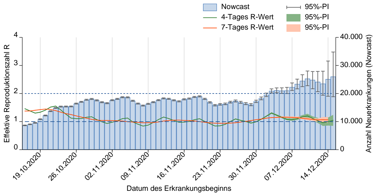
Abbildung 5: Darstellung der geschätzten R-Werte (in grün und orange) in den letzten 60 Tagen, vor dem Hintergrund der durch das Nowcasting geschätzten Fallzahlen nach Erkrankungsbeginn (Stand 19.12.2020, 0:00 Uhr, unter Berücksichtigung der Fälle mit Erkrankungsbeginn bis 15.12.2020).
