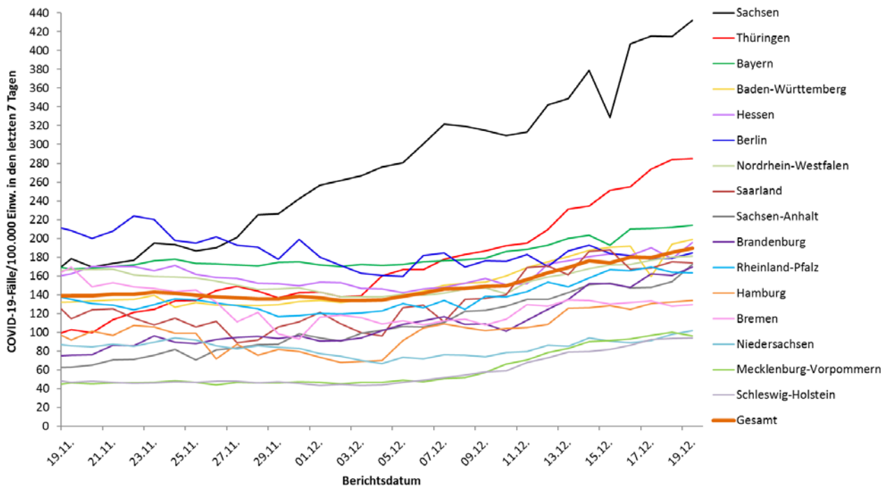
Abbildung 3: Darstellung der übermittelten COVID-19-Fälle/100.000 Einwohner über 7 Tage in Deutschland nach Bundesland (19.12.2020, 0:00 Uhr). In Bundesländern mit vergleichsweise niedrigen Bevölkerungszahlen können auch schon kleinere Anstiege der Fallzahlen zu einer deutlichen Erhöhung der 7-Tage-Inzidenz führen.
