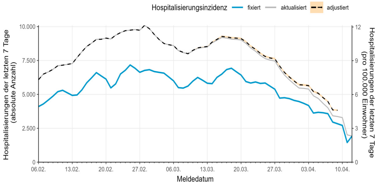
Abbildung 3: Darstellung der hospitalisierten COVID-19-Fälle/100.000 Einwohner über 7 Tage in Deutschland nach Meldedatum (12.04.2023, 0:00 Uhr). Die tagesaktuell berichtete Hospitalisierungsinzidenz (fixiert) wird in blau, mit Berücksichtigung der verzögert berichteten Hospitalisierungen (aktualisiert) in grau dargestellt. Die Schätzung der zu erwartenden Anzahl an verzögert berichteten Hospitalisierungen wird als gestrichelte Linie mit 95%-Prädiktionsintervall (in orange) gezeigt. Die Skalen geben die jeweilige absolute Anzahl (y-Achse, links) und den Anteil pro 100.000 Einw. (y-Achse, rechts) an.
