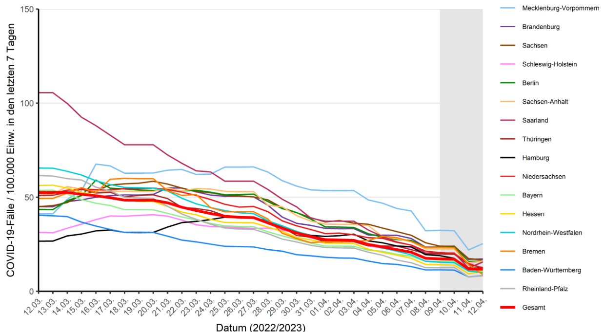
Abbildung 2: Darstellung der übermittelten COVID-19-Fälle/100.000 Einwohner über 7 Tage in Deutschland nach Bundesland und Meldedatum in den Gesundheitsämtern (12.04.2023, 0:00 Uhr). Für den grau markierten Bereich ist in den Folgetagen noch mit nachübermittelten Fällen und damit mit einer Erhöhung der Inzidenz zu rechnen.
