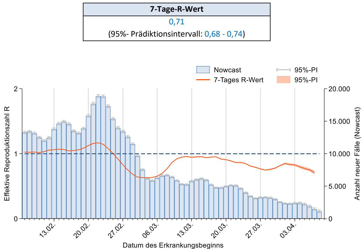
Abbildung 4: Darstellung des geschätzten R-Werts (in orange) in den letzten 60 Tagen, vor dem Hintergrund der durch das Nowcasting geschätzten Fallzahlen nach Erkrankungsbeginn (Stand 12.04.2023, 0:00 Uhr, unter Berücksichtigung der Fälle mit Erkrankungsbeginn bis 08.04.2023).
